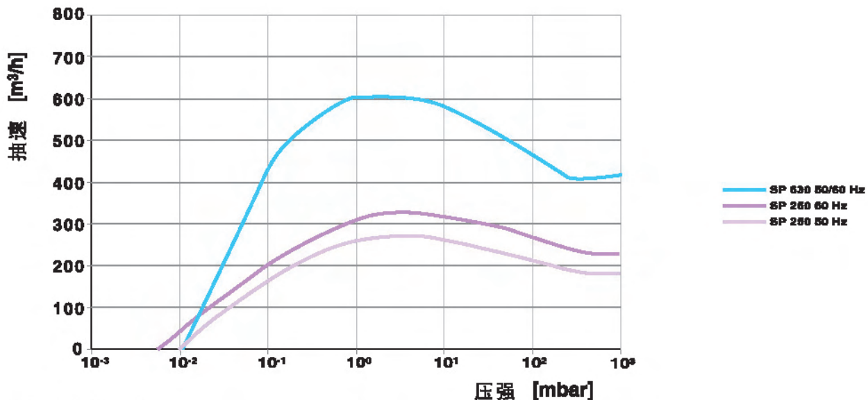
SCREWLINE抽速特性曲线
