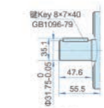
2号轴件 Shaft 2
