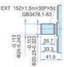
H6号渐开线花键轴件
