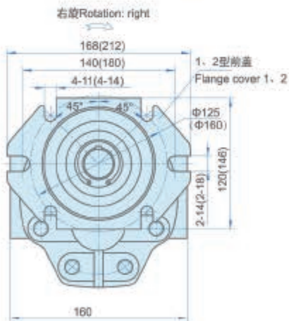
外形尺寸表 Dimension table
